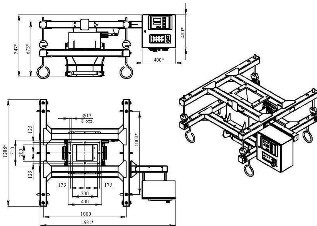
Рис. 1. Габаритно-установочные размеры.
