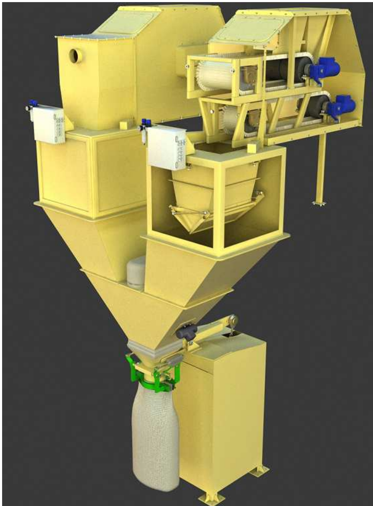
Рис.2. Общий вид.
