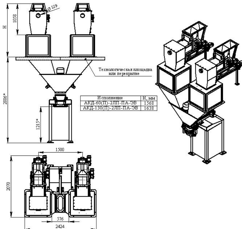
Рис. 1. Габаритно-установочные размеры.
