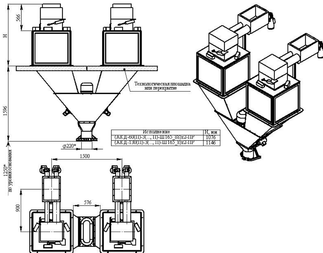
Рис. 1. Габаритно-установочные размеры.
