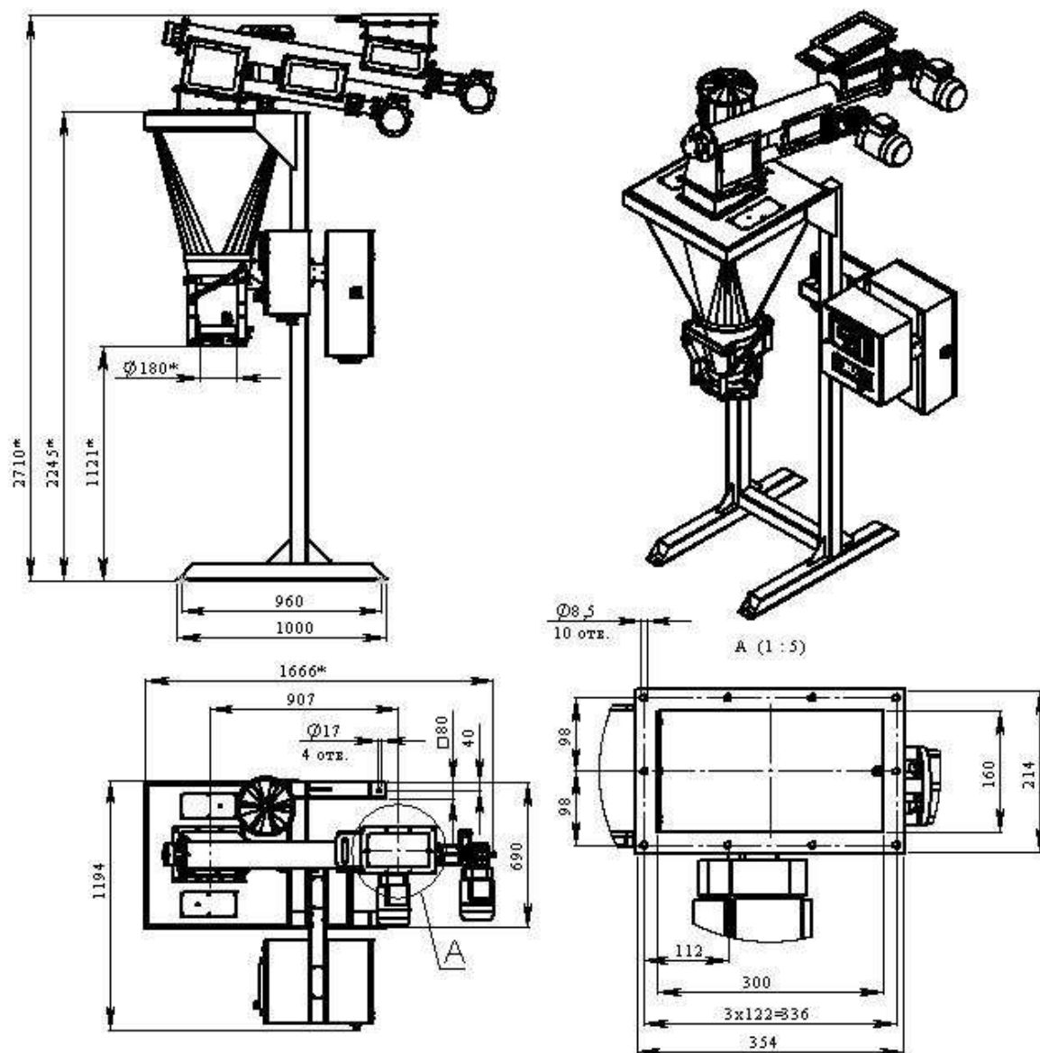
Рис 1. Габаритно-установочные размеры
